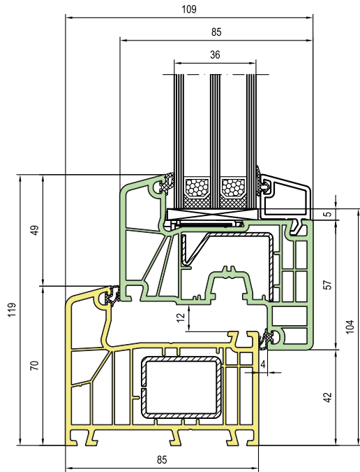
Inåtgående fönster standardkarm och -båge
