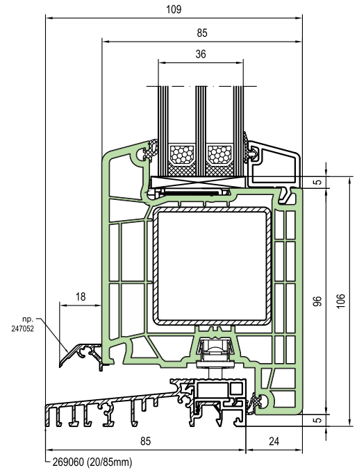
Inåtgående balkongdörr standardbåge och tröskel
